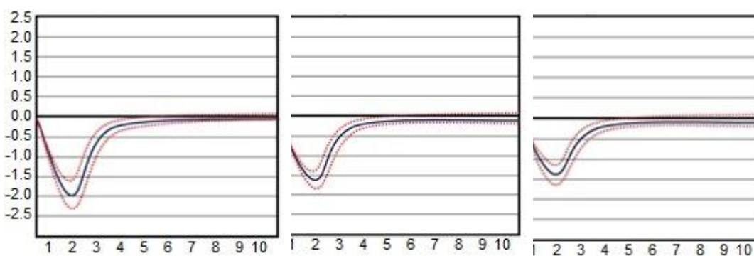
نمودار ۴. واکنش BPR به شوک OLP در سناریو ۱
